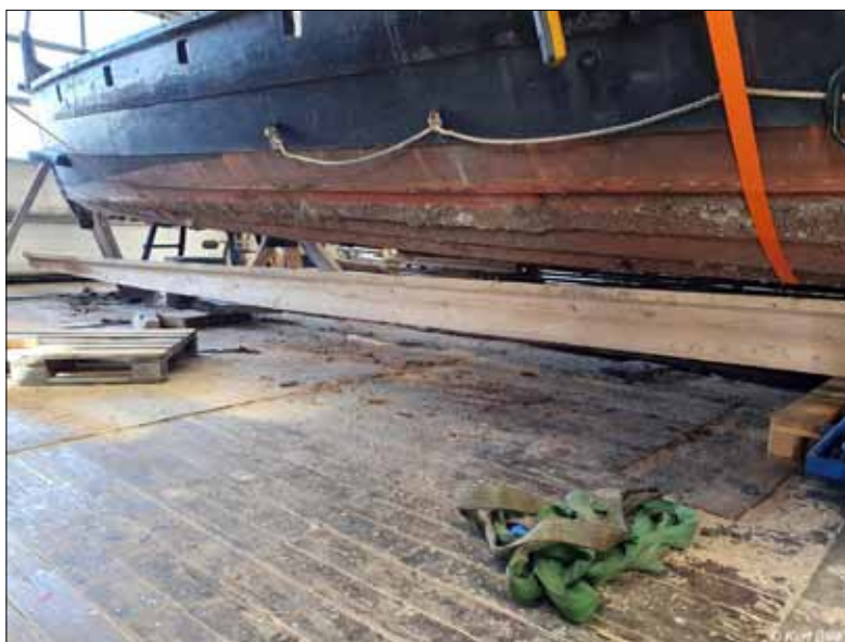
Den gamle køl er fjernet og den nye gøres klar
